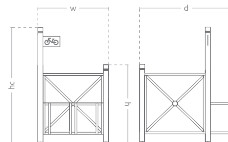
pohled
