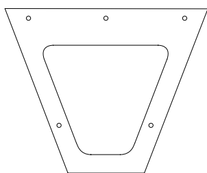
2 Podpěry 11 x
